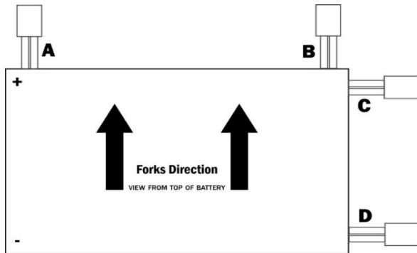
DIRECCIÓN DE LA HORQUILLAS VISTA DESDE LA PARTE SUPERIOR DE LA BATERÍA
